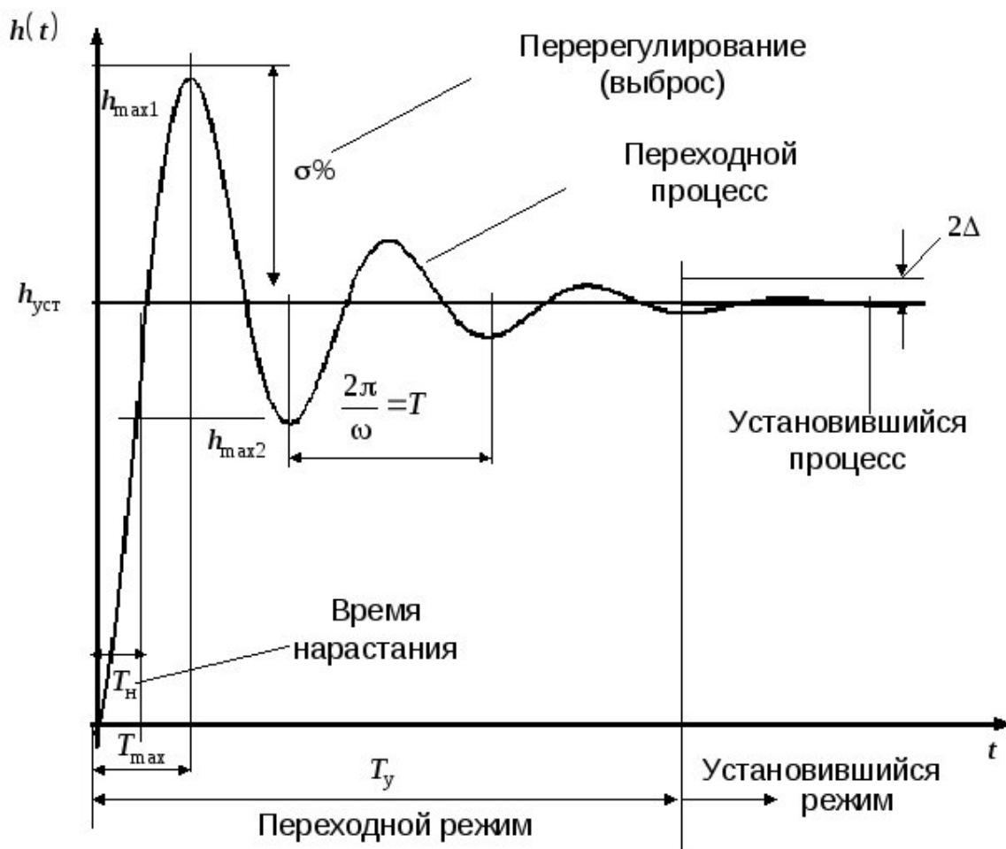
Рис. 1 – Переходная характеристика системы управления
